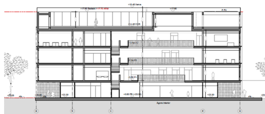
Secció Longitudinal
