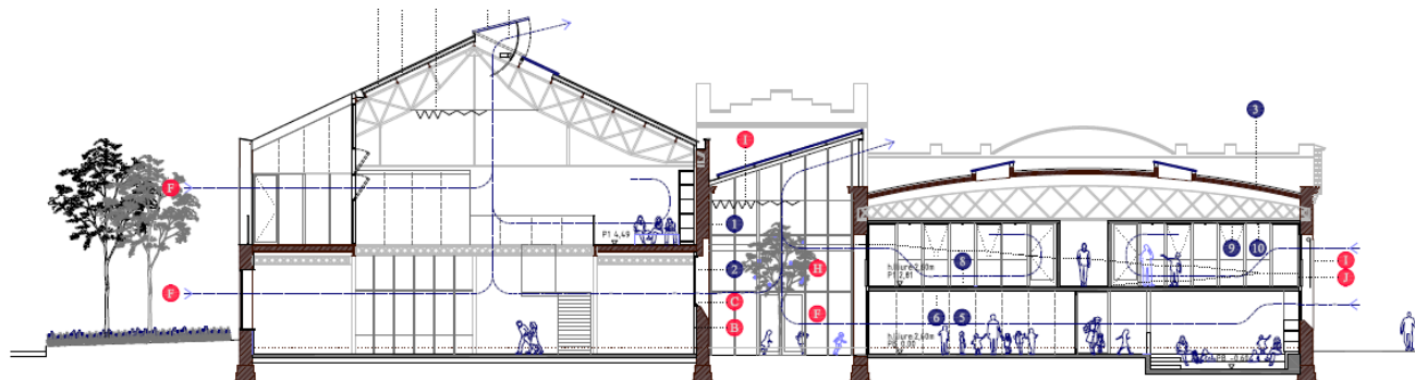
Secció Longitudinal
